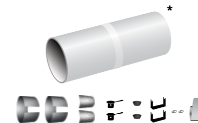
Dvojitě těsněný smrštitelný spoj (FTS DSJ)
